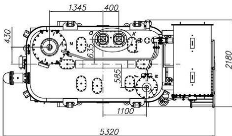
ОЦ-30700/220/Г1 (безвыносной системы охлаждения)
